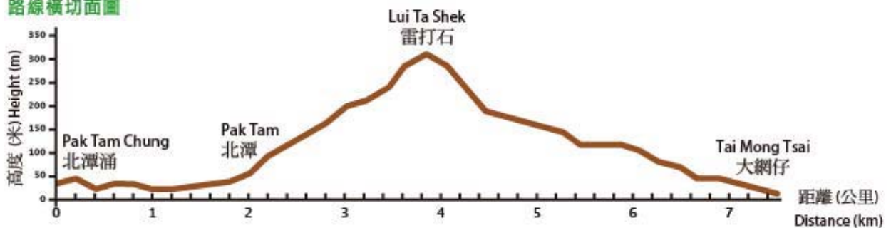
Cross-section 路線橫切面圖
